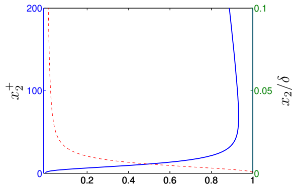
Shear stresses. — : -\rho \overline{v_1' v_2'} / \tau_w ; - - : \mu (\partial \bar{v}_1 / \partial x_2) / \tau_w .
